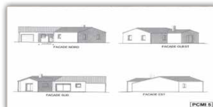
Plan des façades et des toitures.
