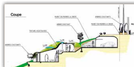
Plan en coupe du terrain et de la construction.
